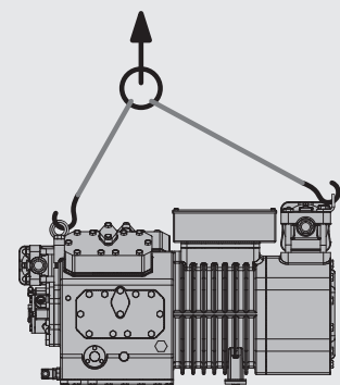
Рис. 1 Подъем компрессора
